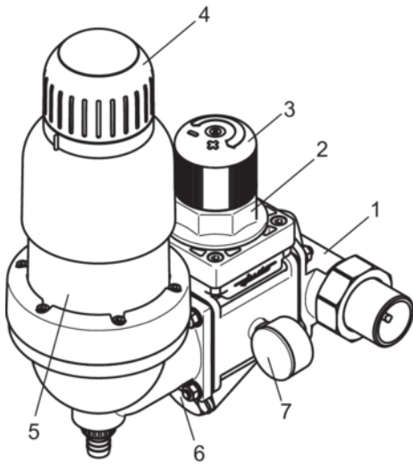
Abbildung 1: Funktionsbeschreibung
