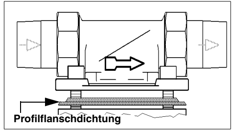
Abb. 3: Einbaudrehflansch
