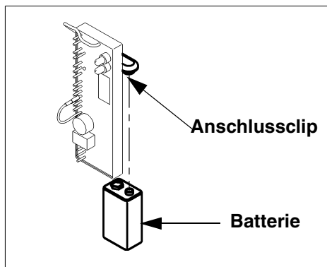
Abb. 12: Batteriewechsel
