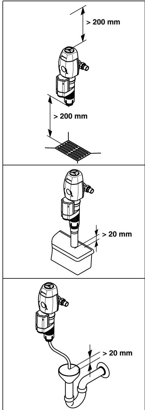
Abb. 6: Ableitungsmöglichkeiten
